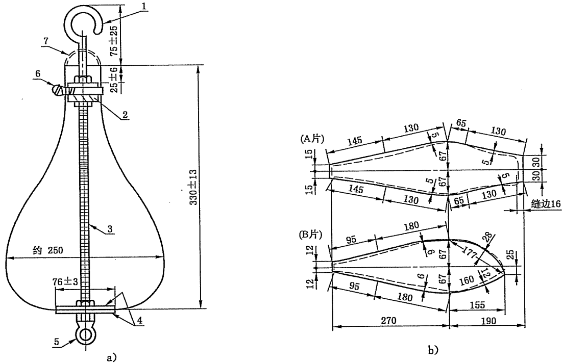
图 C.2 试样框架结构示意图
